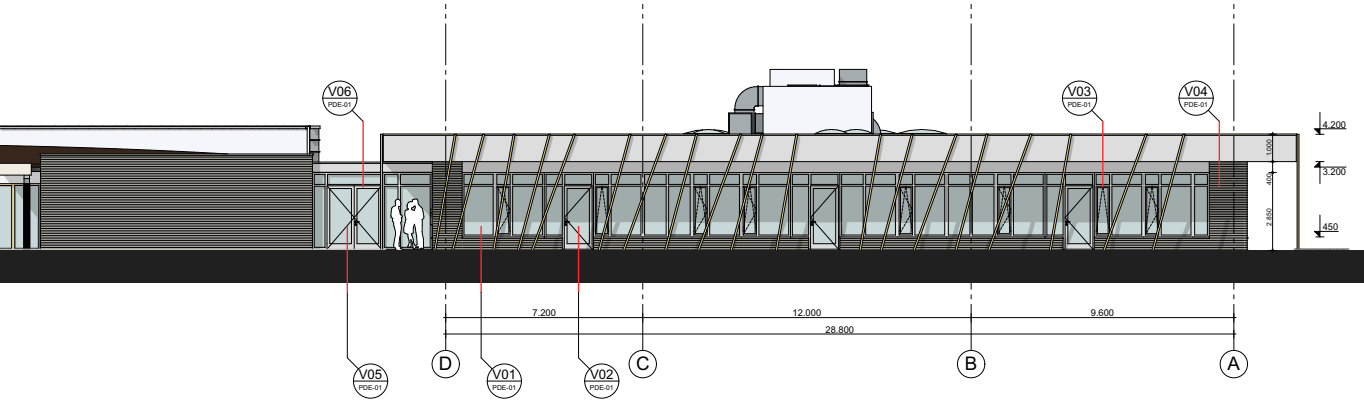
02 PLG-00 zuidwestgevel
